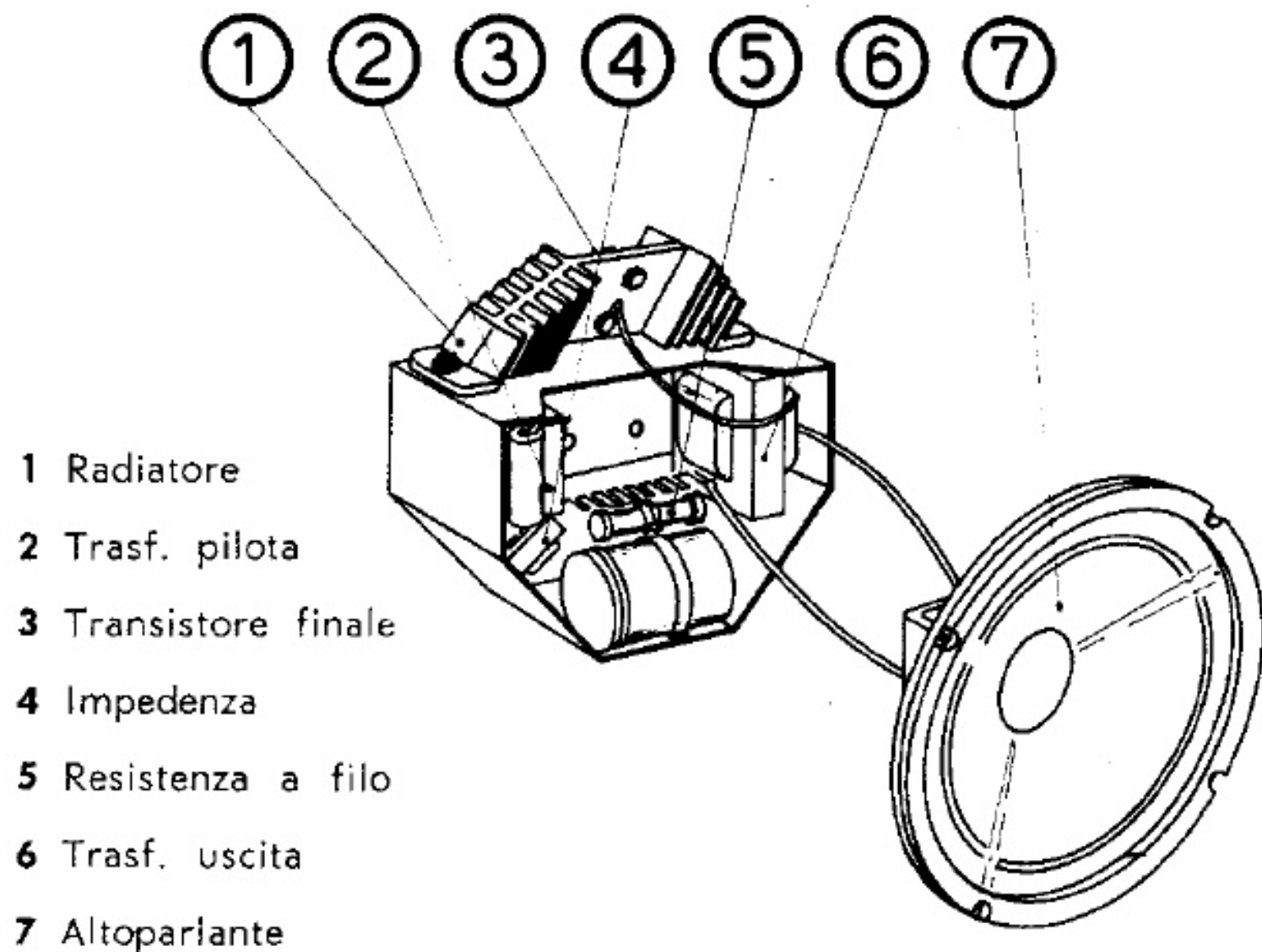
Fig. 3 - Disposizione delle parti principali che compongono il gruppo B 745.
